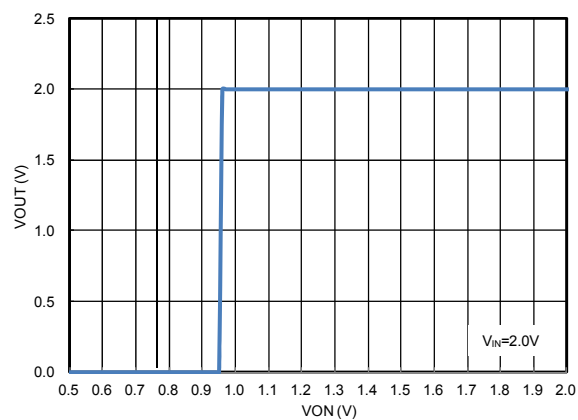
VOUT vs. VON
