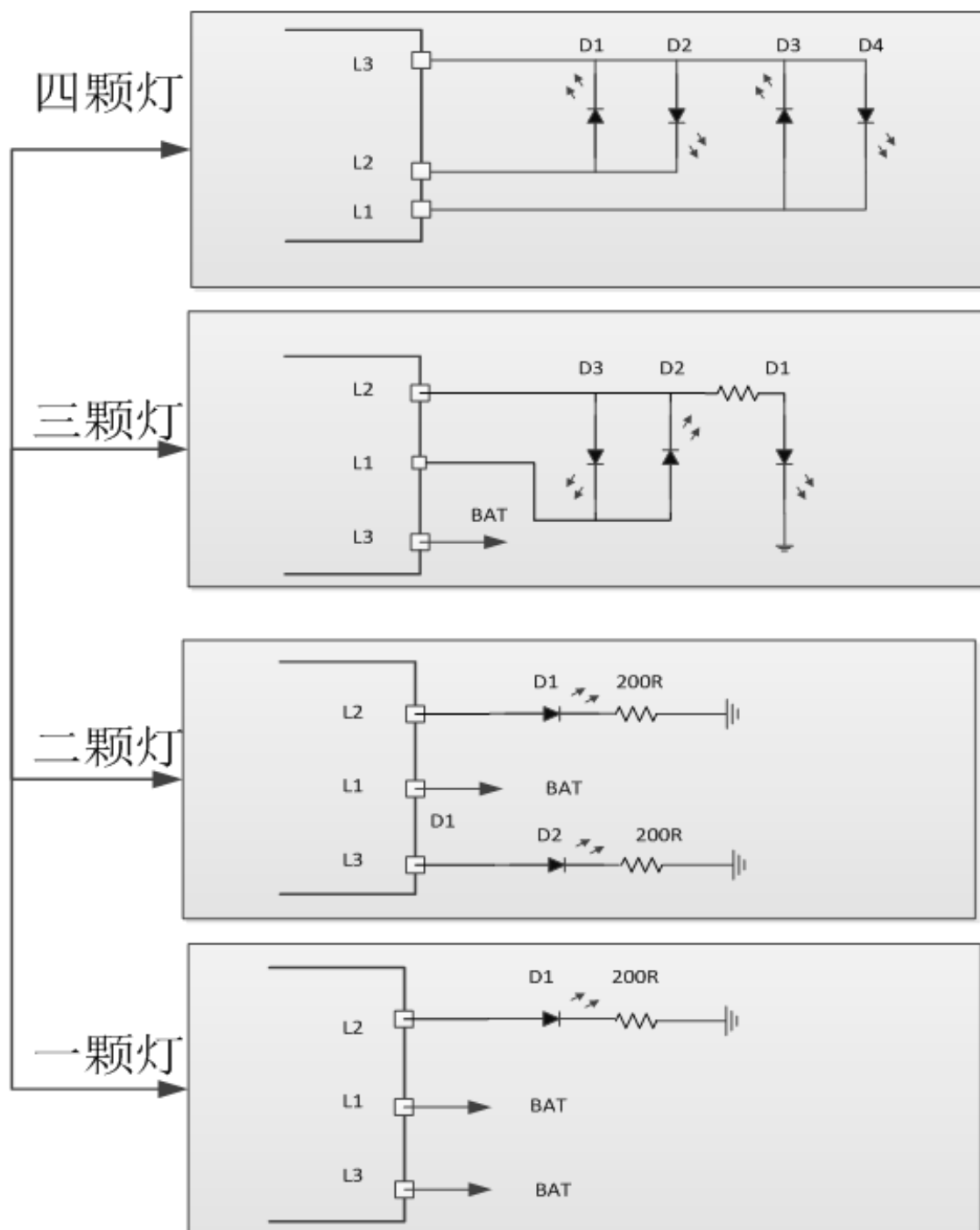
图 5 灯显模式
