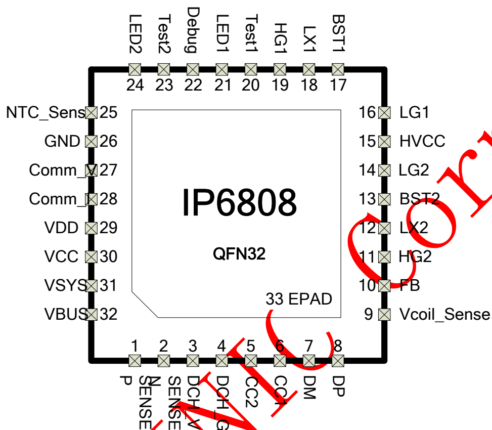
图 2 IP6808 引脚图
